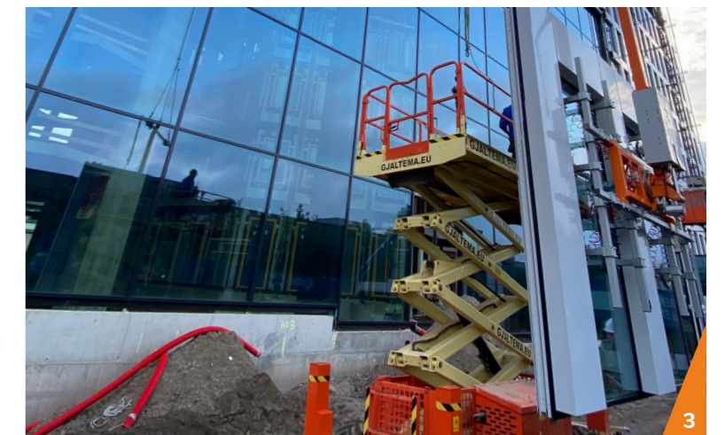
1 Prefab gevelsysteem monteren op project Tripolis Park te Amsterdam 2 Groot formaat ruiten bij gevelbouw van New Amsterdam Court House in Amsterdam 3 Om voorbij de cassettes van het gevelement te komen zijn er afstandhouders van 220 mm gebruikt
