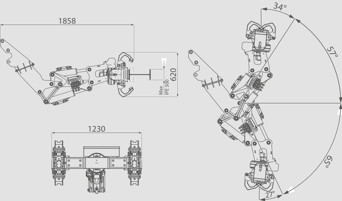
Grabber 500 kg
