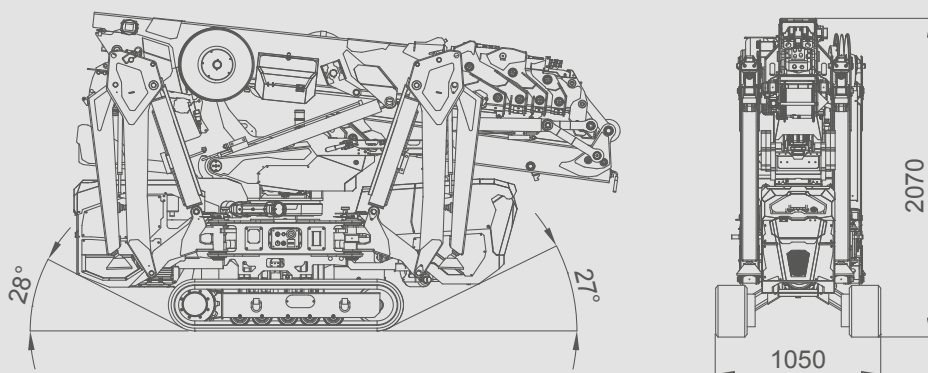
Rupsen verbreed
