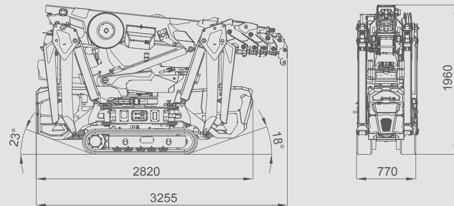
Jib gedemonteerd
