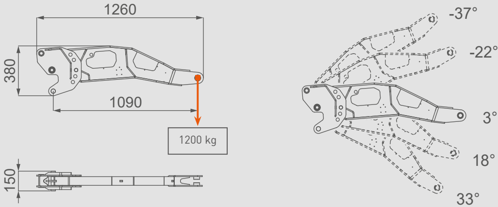
Handjib 1.200 kg
