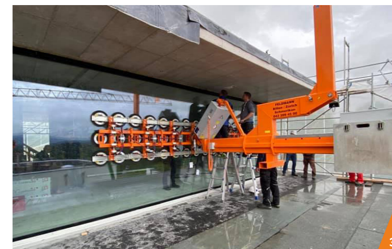
1 Bouwmaterialen aanleveren met behulp van evenaar uitgerust met hijshaak 2 Stalen frame plaatsen op een hoogbouwproject in Engeland 3 Groot formaat ruit plaatsen onder overstek op een project in Zwitserland
