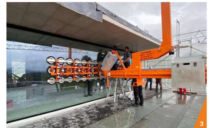
1 Zwaargewicht evenaar met demontabele ballastgewichten van 50,0 kg 2 Dit is bij uitstek de evenaar voor inzetten in de betonbouw 3 Groot formaat ruit plaatsen onder overstek op een project in Zwitserland
