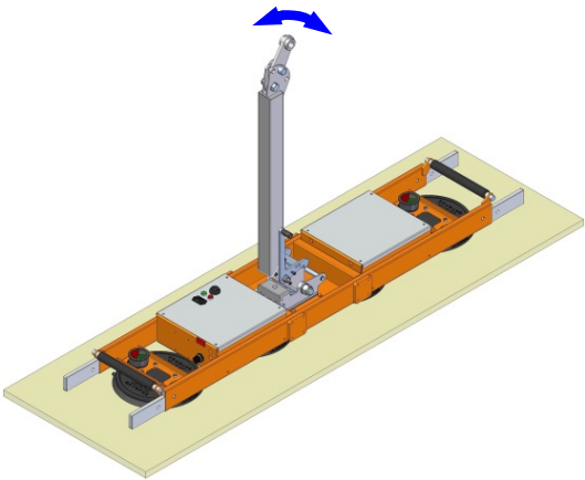
Handmatig 360° roteren Acht vergrendelingsposities
